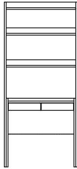
80 デスク W800×D440×H1800 (720) WN ¥134,000+tax Oak ¥120,000+tax
