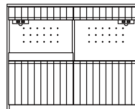
120 キッチンカウンター W1174xD465xH940 家電収納:557×425×360 家電スライド収納:515×425×295 WN ¥203,500 (¥185,000+tax) Oak ¥187,000 (¥170,000+tax) スライドカウンターは左右に付け替え可能。
