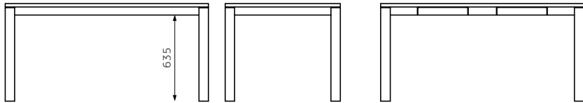
120~200 ダイニングテーブル・脚A~C W1200~2000xD750~900xH720
