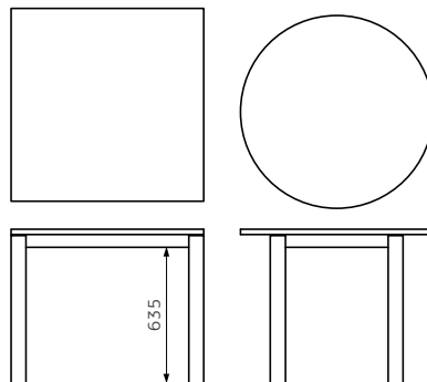
90~120 スクエア/ラウンドテーブル・脚A~C W900~1200xD900~1200xH720
